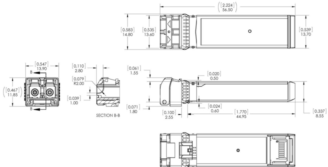
FTLF8532P4BCV
